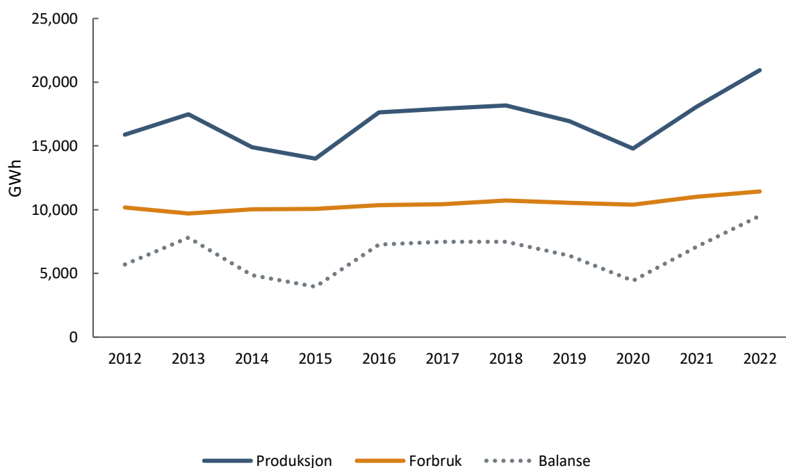
Figur 4-4 Produksjon, forbruk og energibalansen for kraft i Nordland, GWh, 2012-2022. Figuren viser at Nordland hadde et overskudd på over 9 000 GWh (9 TWh) i 2022, der produksjonen lå på omtrent 20 000 GWh (20 TWh) og forbruket på 11 000 GWh (11 TWh). Produksjonen er realisert produksjon, og derfor varierer mengden fra år til år, grunnet sesongvariasjoner, som vær, nedbør og vindforhold.
